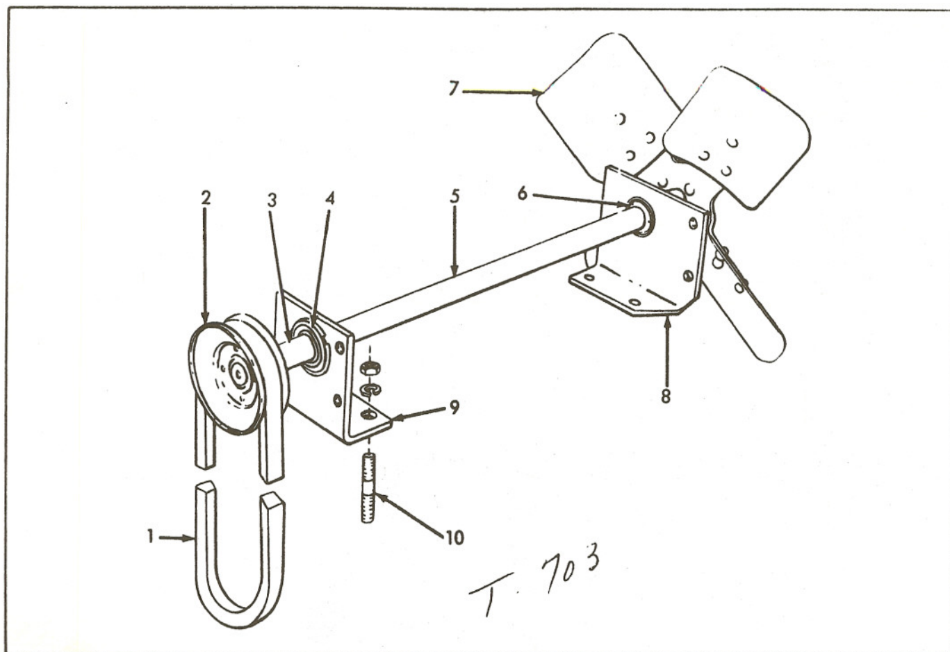
FAN
