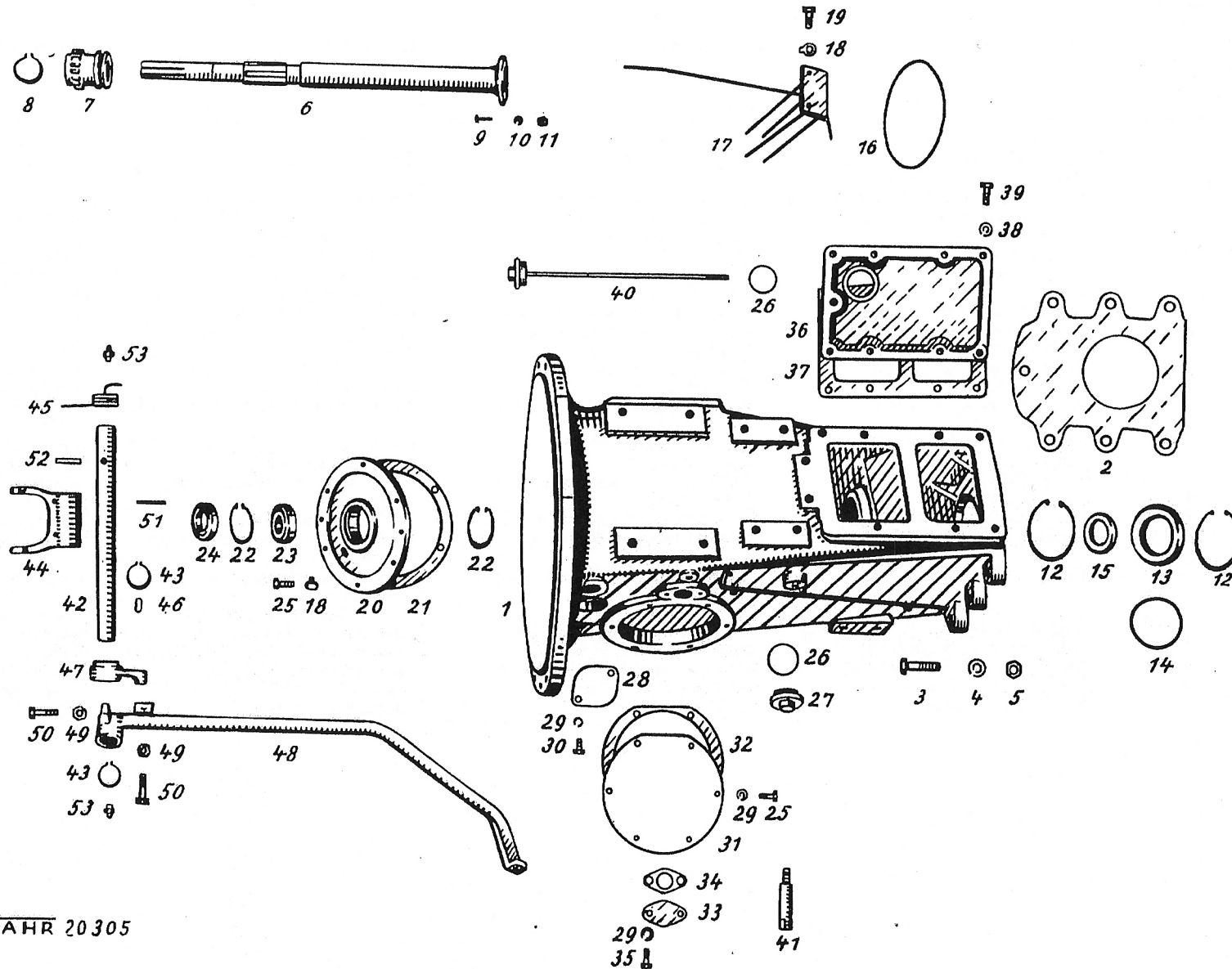
Caja abridada de embrague
