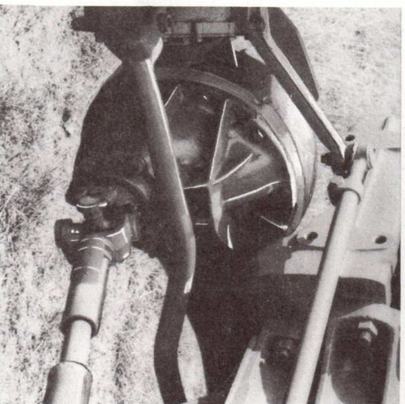
Entretien par arbre coulissant cannelé et joints de cardans.
