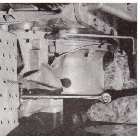
Un levier à portée de la main commande la prise de mouvement.
