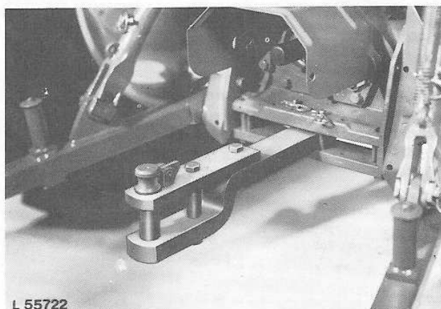
Barre d'attelage avec chape
