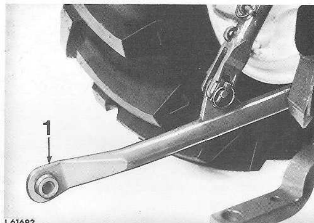
1 Barres de traction réversibles pour outils portés des catégories I et II
