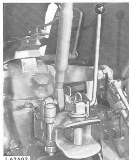
Chape d'attelage en position d'utilisation
