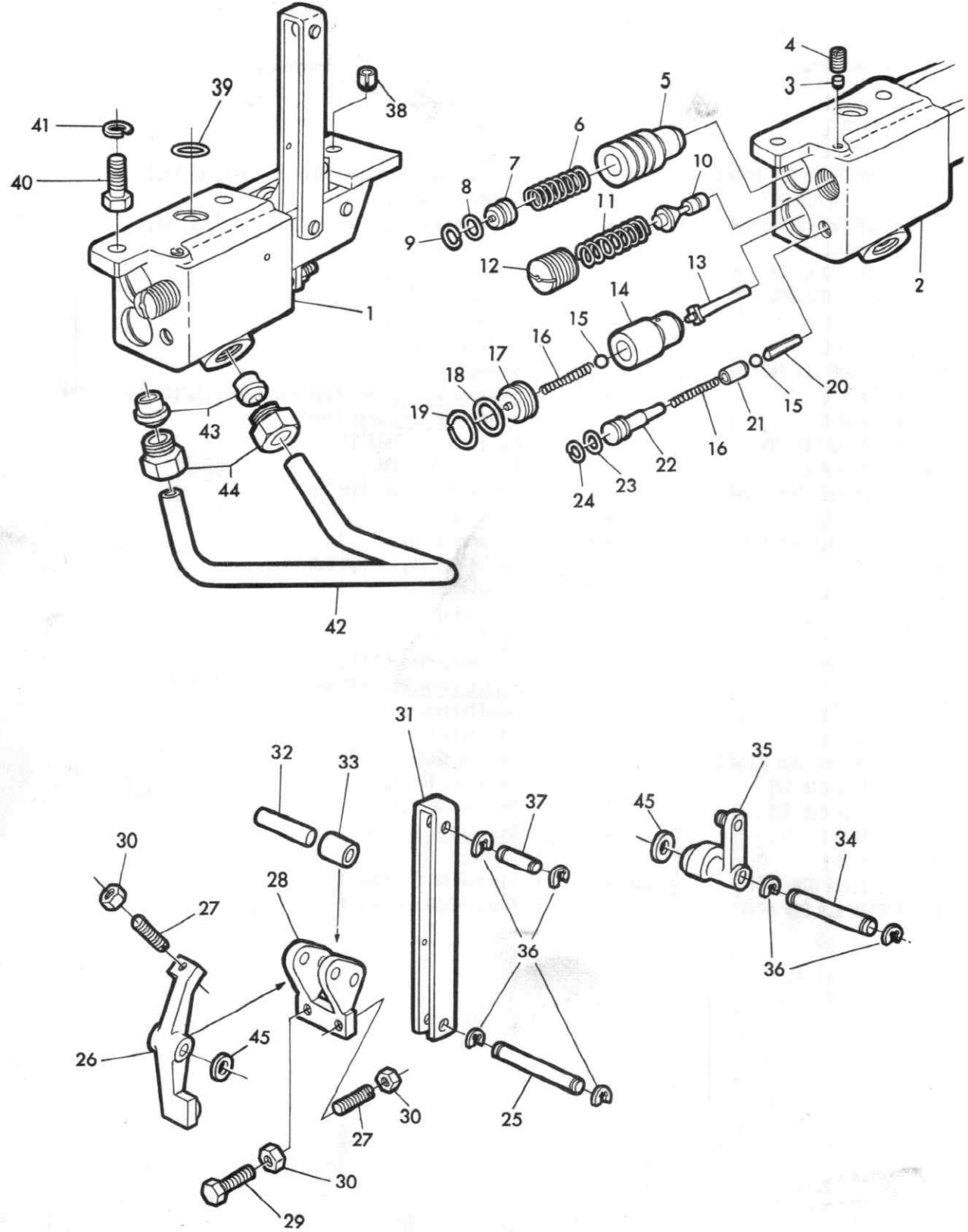
Kraftheber-Steuerung (Bild 2) Control Valve (Fig. 2) Distributeur de relevage hydraulique (ill. 2)
