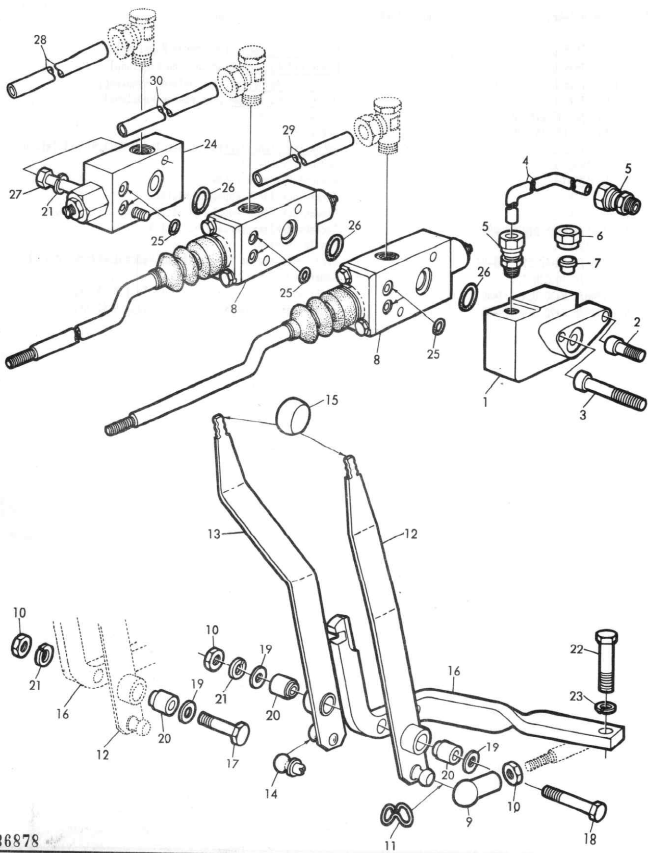
Zusatzsteuergerät (Bild 1) Control Valve (Fig. 1) Dispositif de commande (ill. 1)
