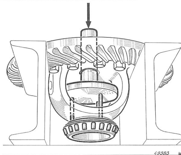
Éclaté du différentiel.
