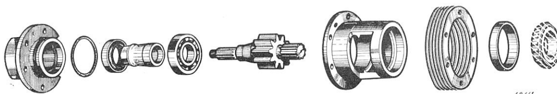
Éclaté arbre de différentiel.
