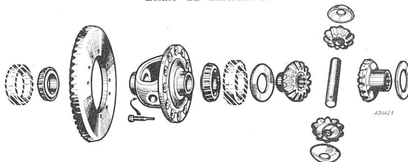
Éclaté du différentiel.
